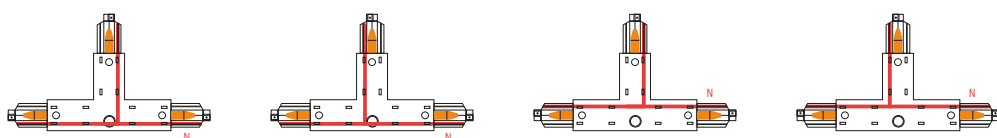
Т-образное соединение (правое внутреннее, правое внешнее, левое внутреннее, левое внешнее)
